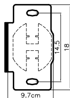
MP18 Winkelgrundplatte: Standard (ab 10 cm Mauerbreite)
