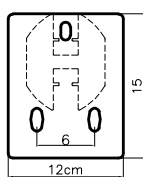
MP17.1 Grundplatte: Bündig (ab 15 cm Mauerbreite)
