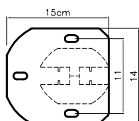
MP8 Grundplatte: bündig längs
