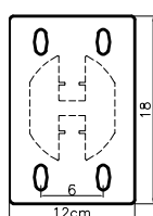
MP17 Grundplatte: Standard (ab 15 cm Mauerbreite)
