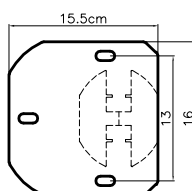
MP9 Grundplatte: bündig quer
