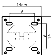
MP11 Grundplatte: Nivillierschrauben
