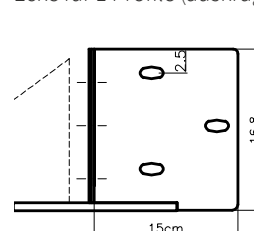
MP19.3 Wandeckplatte flach: Ecke für 1 Profile (auskragend)
