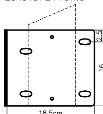
MP19.2 Wandeckplatte flach: Ecke für 2 Profile
