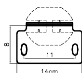
MP5 Winkelgrundplatte: Frontprofil
