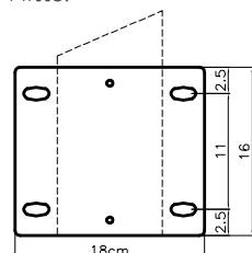
MP19 Wandplatte flach: Mittel
