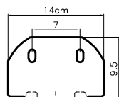
MP8 Grundplatte: bündig längs
