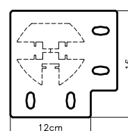
MP18.1 Winkelgrundplatte: bündig, rechts (ab 10 cm Mauerbreite)
