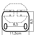
MP6 Winkelgrundplatte: Frontprofil
