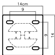
MP1 Grundplatte: Standard Verstärkte Platten: MP23 / MP28
