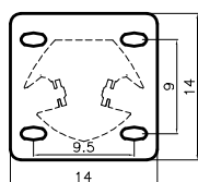
MP22 Grundplatte flach: Spezialwinkelprofil
