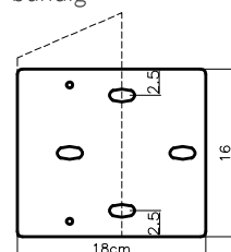
MP19.1 Wandplatte flach: bündig
