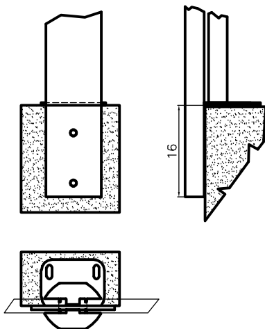
Frontmontage mit Grundplatte
