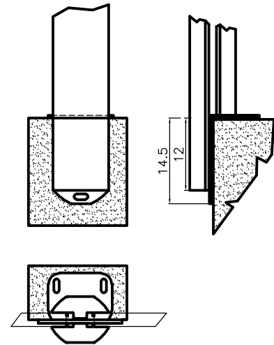
Frontmontage mit Winkelgrundplatte
