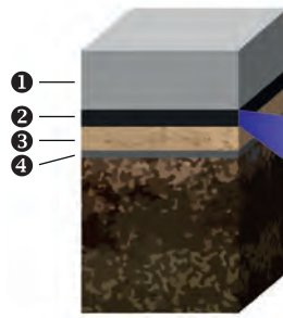
Aufbau BERA® Stable Pave
